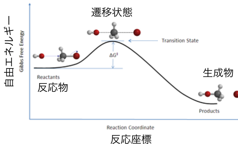
図 反応座標と遷移状態
